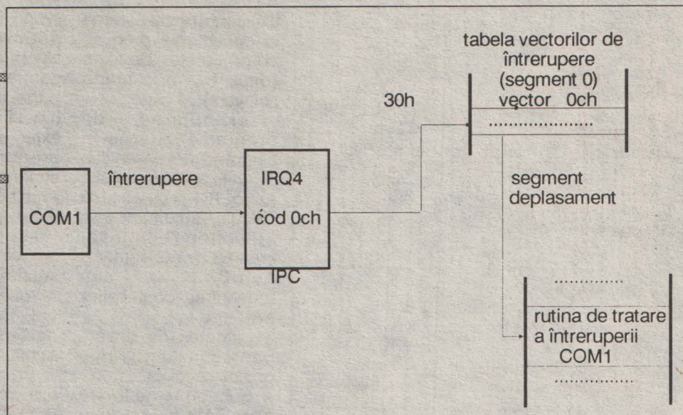
Fig.2. Modul de pointare a vectorilor de întrerupere la rutinele corespunzătoare perifericelor.
